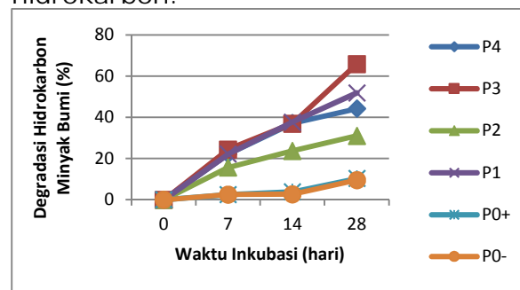
Gambar 1. Degradasi minyak bumi selama inkubasi 28 hari.
