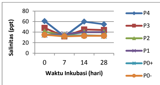
Gambar 9. Nilai salinitas seluruh perlakuan selama waktu inkubasi 28 hari.
