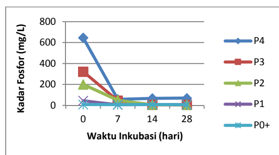
Gambar 5. Kadar fosfor seluruh perlakuan selama waktu inkubasi 28 hari.
