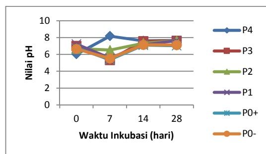
Gambar 8. Nilai pH selama waktu inkubasi 28 hari.
