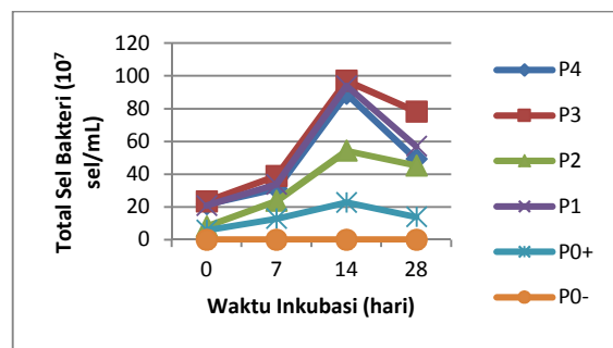
Gambar 2. Jumlah total sel bakteri selama waktu inkubasi 28 hari.
