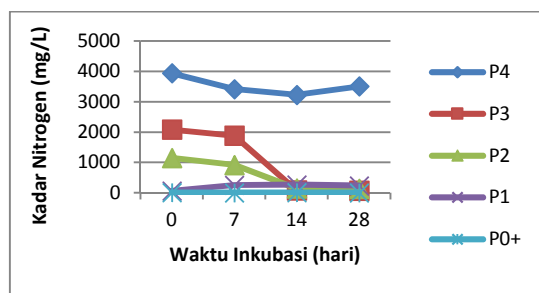
Gambar 4. Kadar nitrogen seluruh perlakuan selama waktu inkubasi 28 hari.
