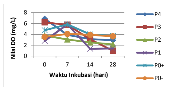
Gambar 6. Nilai oksigen terlarut seluruh perlakuan selama waktu inkubasi 28 hari.
