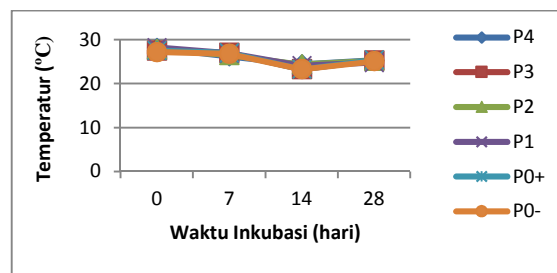
Gambar 7. Nilai temperatur seluruh perlakuan selama waktu inkubasi 28 hari.
