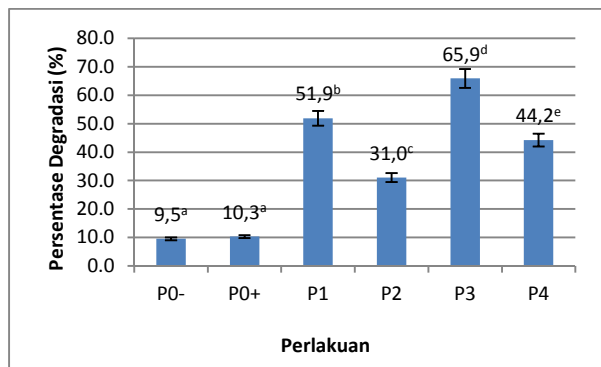
Gambar 3. Persentase degradasi minyak bumi selama 28 hari inkubasi. Huruf yang sama pada persentase degradasi menunjukkan berbeda tidak nyata.
