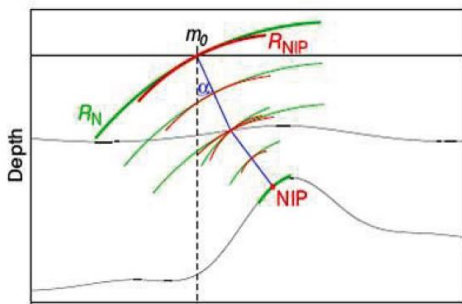
Gambar 3 Curvature gelombang normal (hijau) dan Curvature gelombang NIP (merah) (Duvencek, 2004)
