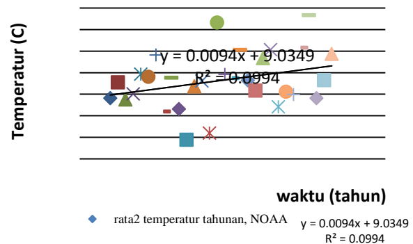
Gambar 4. Grafik temperatur udara daerah Kabupaten Semarang periode 30 tahun (1984-2013)
