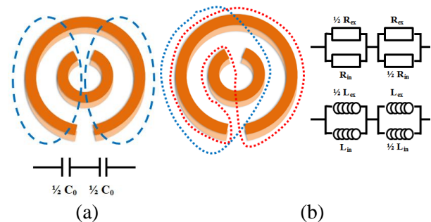
Gambar 4.2 Rangkaian ekuivalen dari SRR (a) kapasitansi efektif, (b) induktivitas, dan resistivitas efektif
