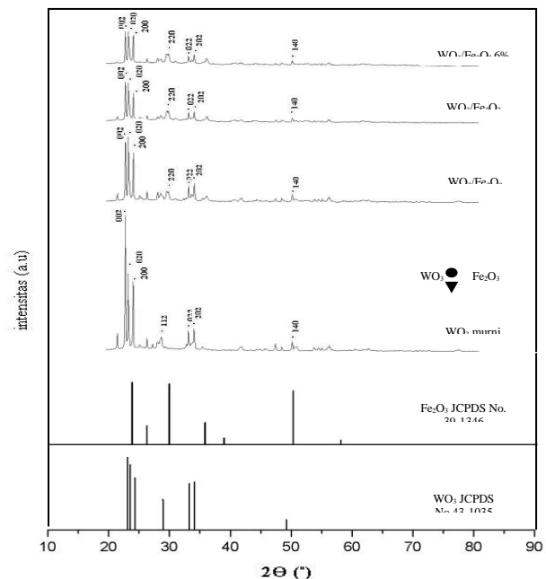
Gambar 6. Pola XRD film WO 3 /Fe 2 O 3
