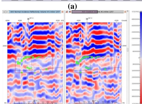
Gambar 5 (a) Krosplot antara intercept (sumbu-x) dan gradient (sumbu-y) pada sumur DBT-12 dan (b) Penampang intercept (kiri) dan gradient (kanan) hasil krosplot yang ditandai dengan warna hijau yang berada disekitar CGL-B
