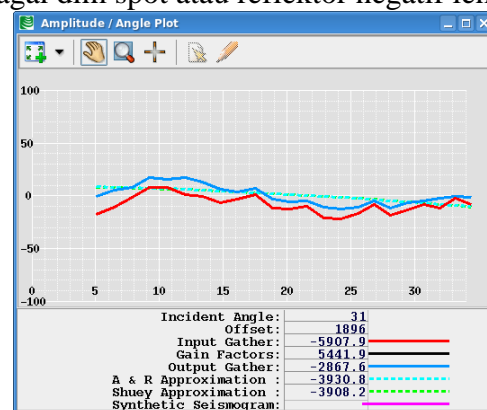
Gambar 4 Grafik antara amplitudo dengan sudut datang di sekitar sumur DBT-12 horizon CGL-B bottom
