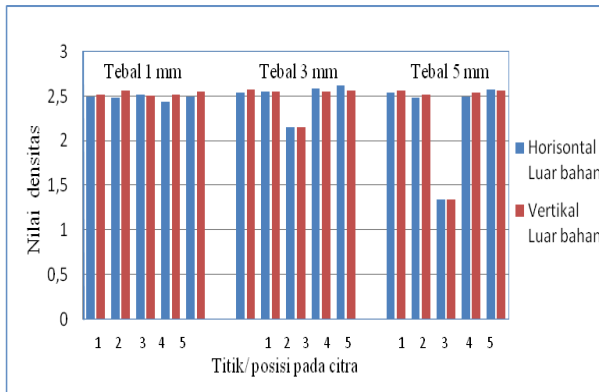
Gambar 11. Perbandingan nilai densitas citra antara grid horisontal dan vertikal posisi luar bahan aluminium
