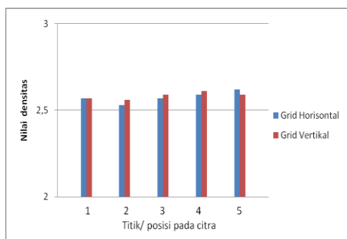
Gambar 9. Nilai densitas citra menggunakan grid bergerak
