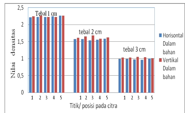
Gambar 12. Perbandingan nilai densitas citra antara grid horisontal dan vertikal dalam bahan akrilik.
