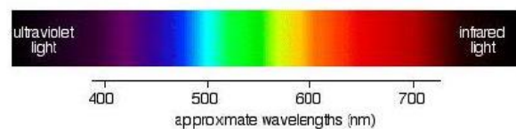
Gambar 2.1 Spektrum cahaya tampak, menunjukkan interval panjang gelombang untuk berbagai warna [4]
