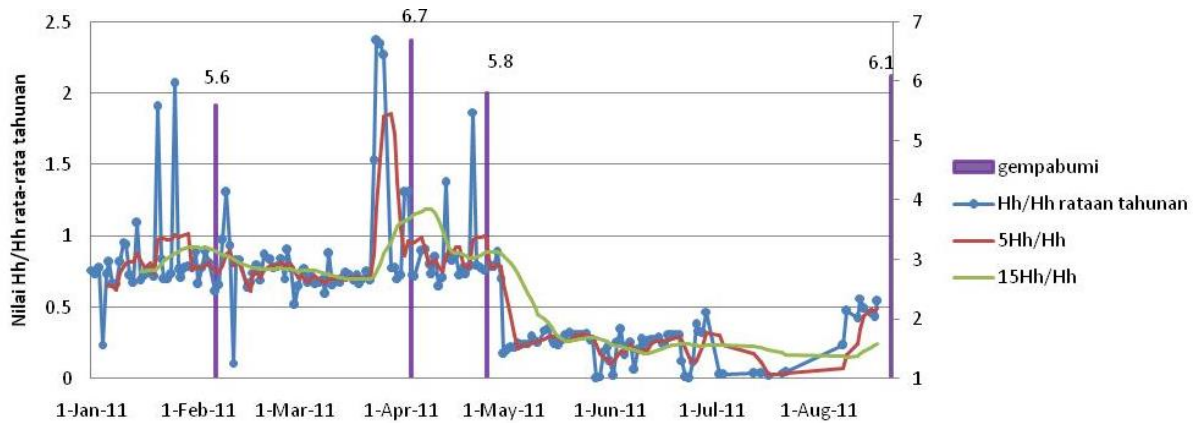
Gambar 4.2. Plot garis warna biru adalah rasio polarisasi variasi magnetik komponen horizontal ( H_h ) terhadap rata-rata tahunan ( Annual Mean ) / ( one year average ). Plot garis warna merah dan hijau adalah rata-rata ( running average )
