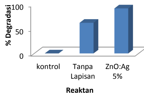
Gambar 6 Persentase degradasi konsentrasi zat warna methylene blue pada fotodegradasi 6 jam.
