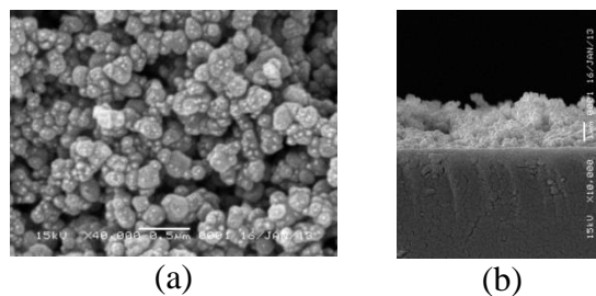
Gambar 4. Citra SEM lapisan tipis \text{TiO}_2 (a) permukaan (b) penampang lintang
