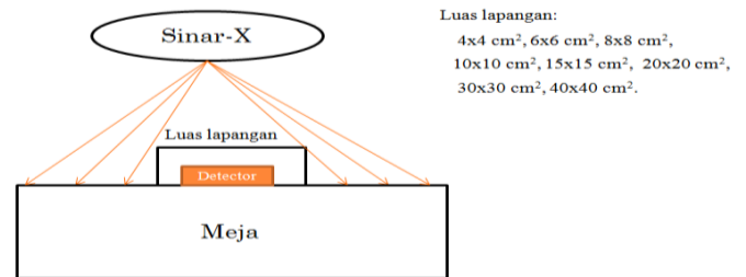
Gambar 3. Diagram blok untuk variasi luas lapangan sinar-X
