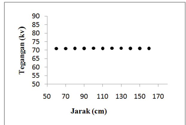
Gambar 6 Grafik tegangan terukur terhadap perubahan jarak MPD-sumber sinar-X.
