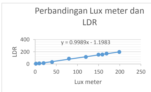
Gambar 13. Perbandingan Lux meter dan sensor LDR
