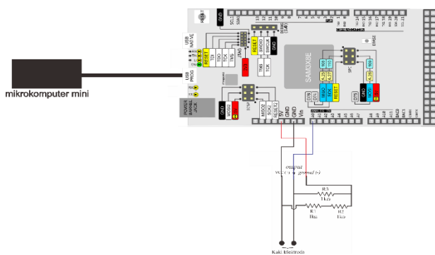
Gambar 2. Rangkaian akuisisi sensor
