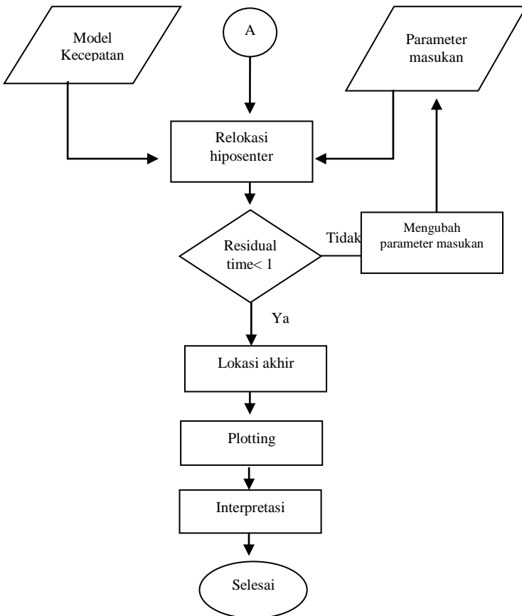
Gambar 7. Diagram alir relokasi hiposenter
