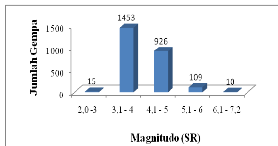
Gambar 10. Grafik distribusi antara jumlah gempa dan magnitudo dari tahun 2004 sampai 2011 sebelum relokasi
