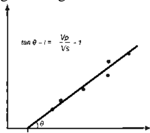
Gambar 3. Grafik Wadati
